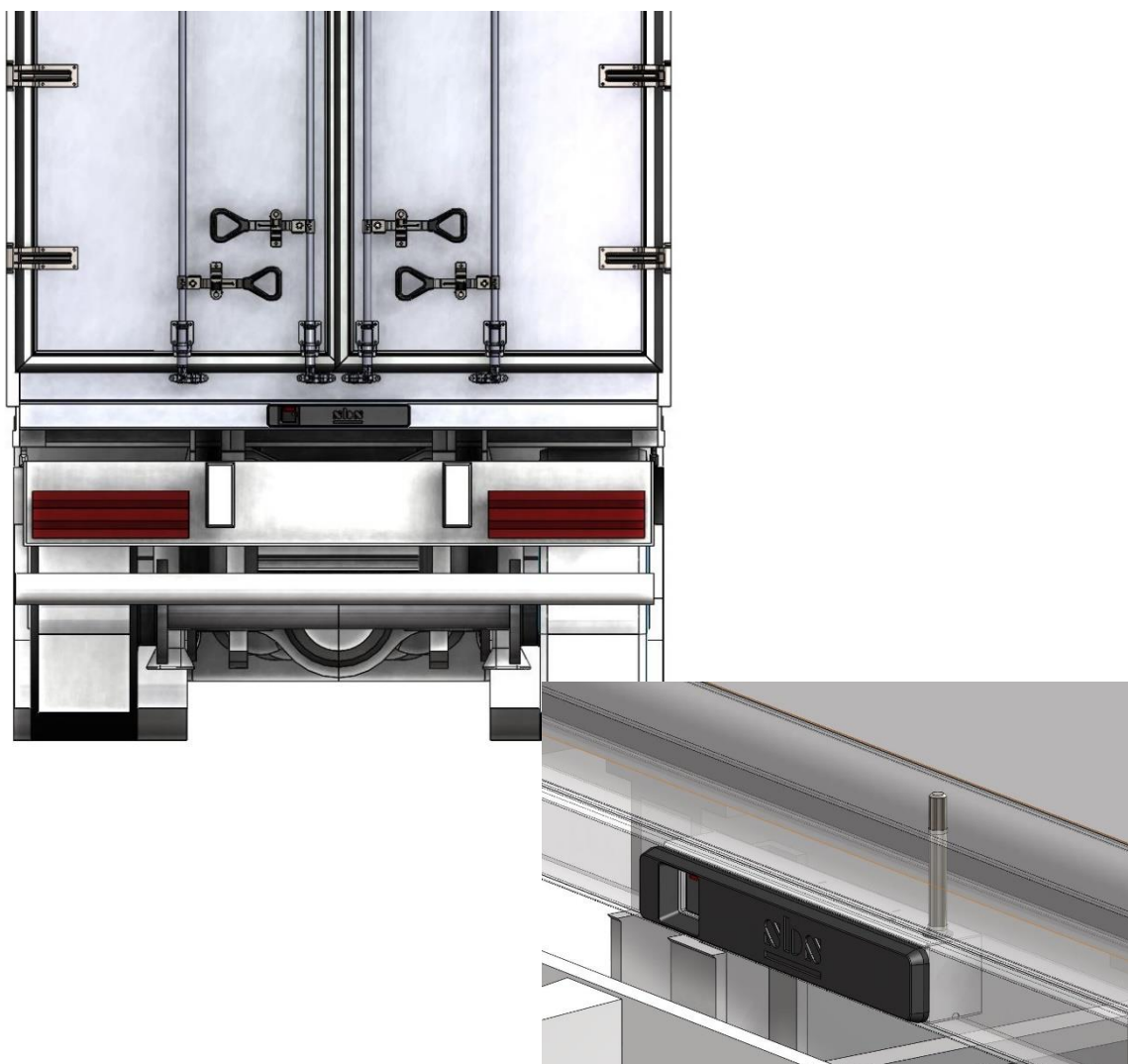
Fot. 1: Schemat SBS Lock-25 – montowany od dołu ramy naczepy. Główny panel widoczny pod linią drzwi. Trzpień blokujący drzwi prawe wysuwany od dołu.
